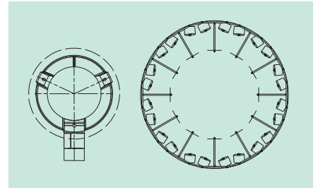
Rundgatter mit oder ohne Blaseinrichtung. Circular creel with or without blowing device.
